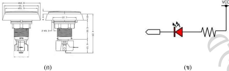
รูปที่ 7 (ก) ปุ่มเกมส์ที่มีหลอดไฟ LED และสวิตช์ ("Large Arcade Button with LED - 60mm Red,") (ข) วงจรการต่อหลอดไฟ LED
